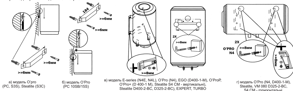
Рис. 4. Кріплення ЕВАД до стіни
