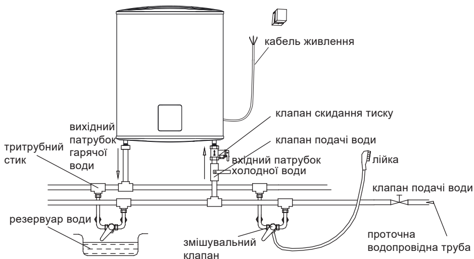
↑ ВЕРТИКАЛЬНЕ ВСТАНОВЛЕННЯ
