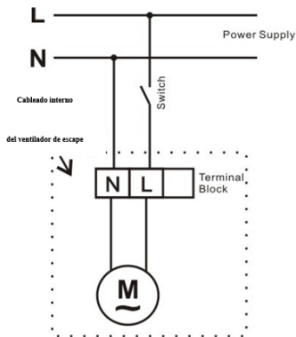
Conexión de cableado estándar
