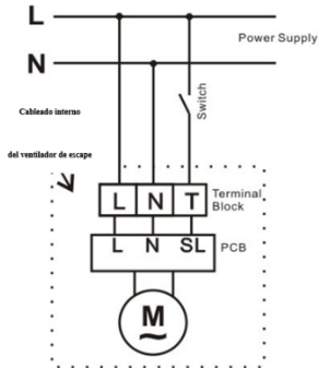
cableado de humedad
