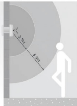
Suprafata de detectare a prezentei
